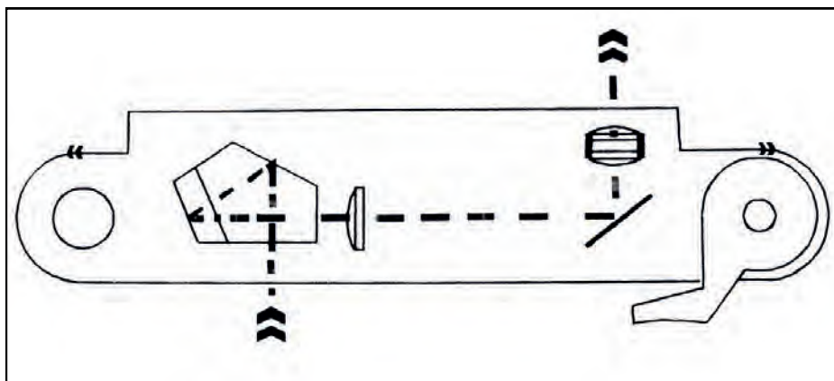
Tegning af afstandsmåleren i Diax-Reflex. Grafik Hans Grether.
